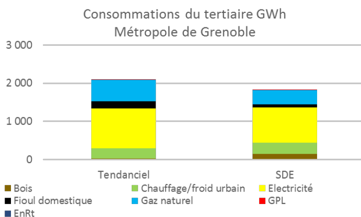
Figure 93 - Répartition des consommations du tertiaire en GWh au niveau de la Métropole de Grenoble en application du tendanciel et Schéma Directeur des Energies par type d'énergie
