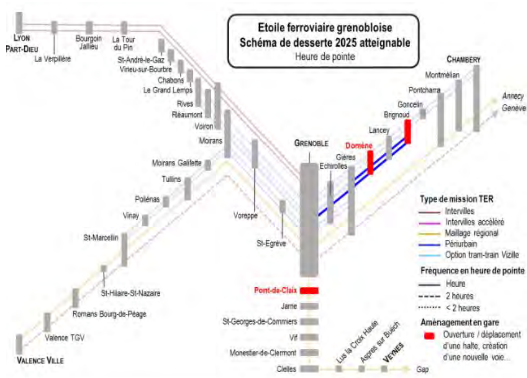
Figure 80 : Projet Étoile Ferroviaire (Source : AURG)
