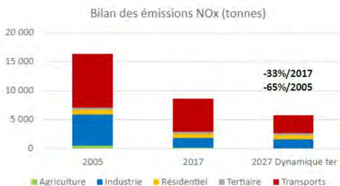
Figure 97 : Bilan des émissions de NOx sur le territoire du PPA3 de Grenoble
