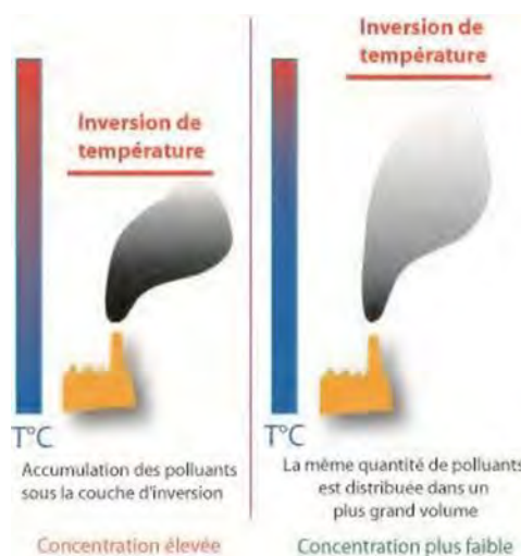
Figure 44 : Inversion de température (Source : Atmo AURA)
