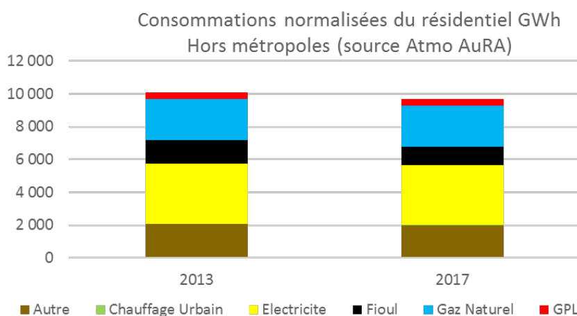
Figure 92 - Répartition des consommations normalisées du résidentiel en GWh en dehors de la Métropole de Grenoble 2013 et 2017 par type d'énergie
