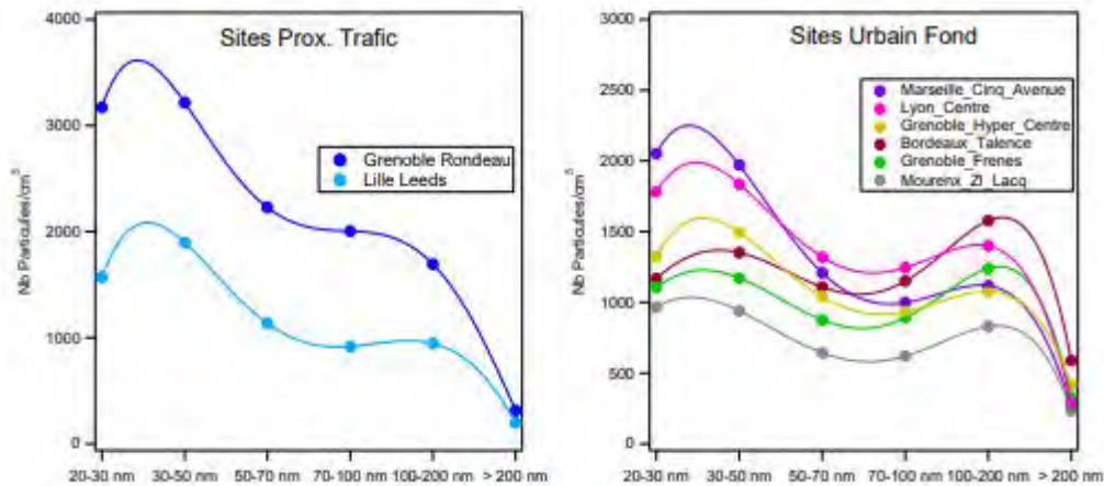
Figure 66 : Distribution granulométrique moyenne des PUF par site [Source : Atmo AURA]
