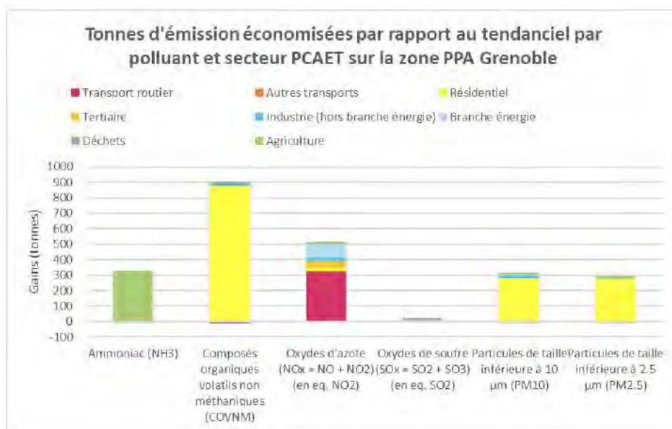
Figure 104 – Réductions d'émission par rapport au tendanciel par polluant et secteur PCAET sur la zone PPA Grenoble
