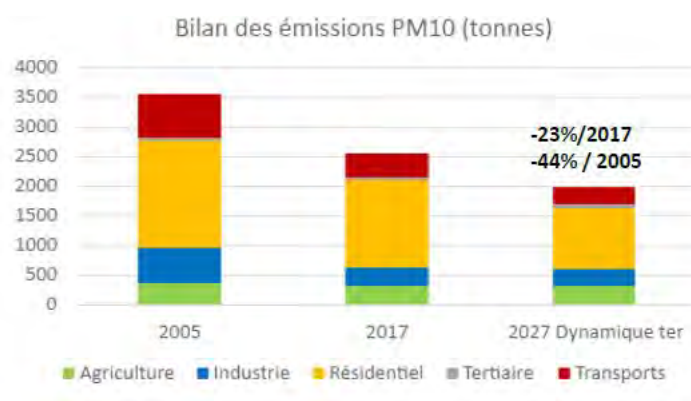
Figure 99 : Bilan des émissions de PM 10 sur le territoire du PPA3 de Grenoble
